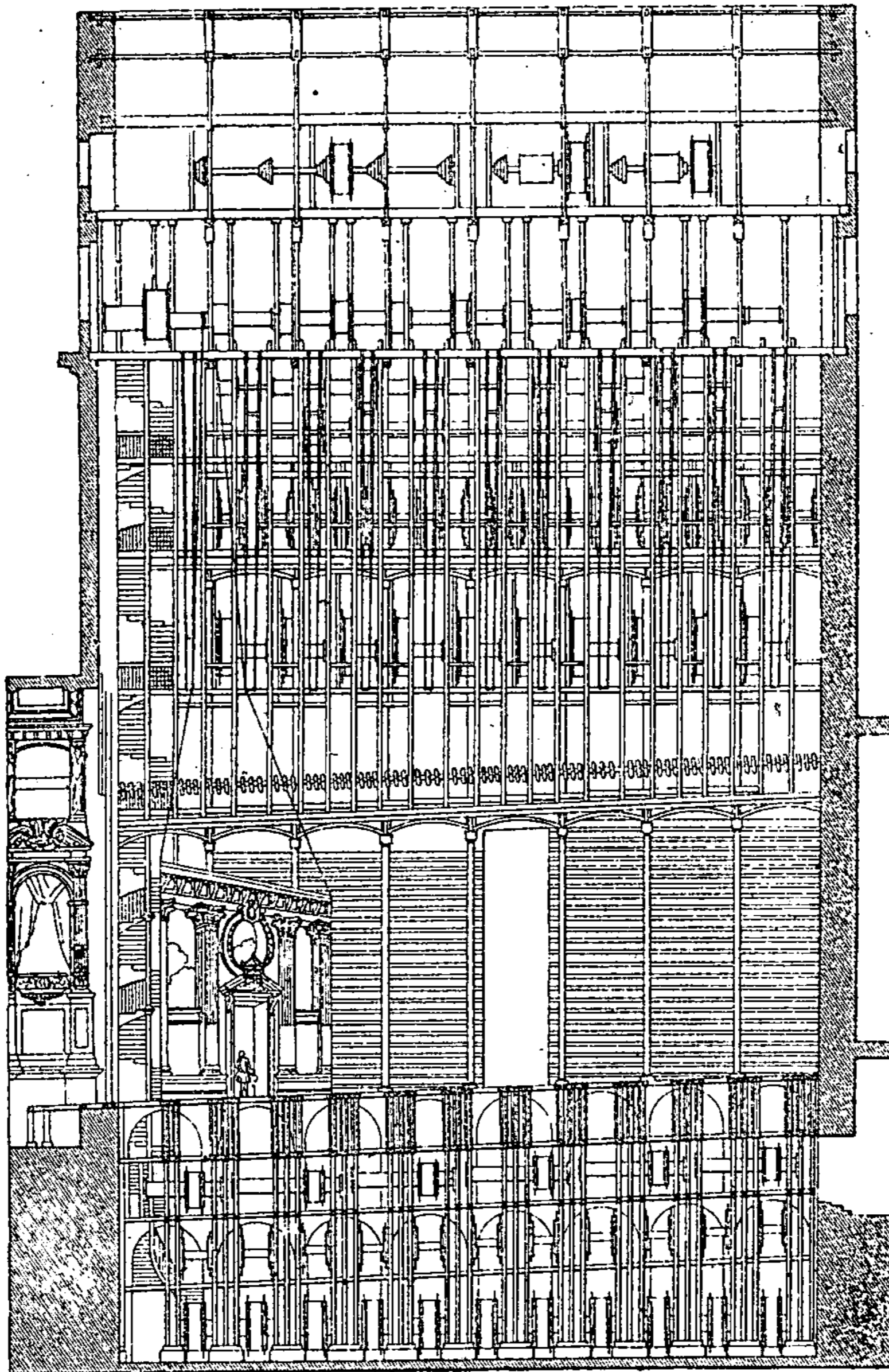
Fig. 2. — Coupe longitudinale d'un théâtre, plafond équipé.
