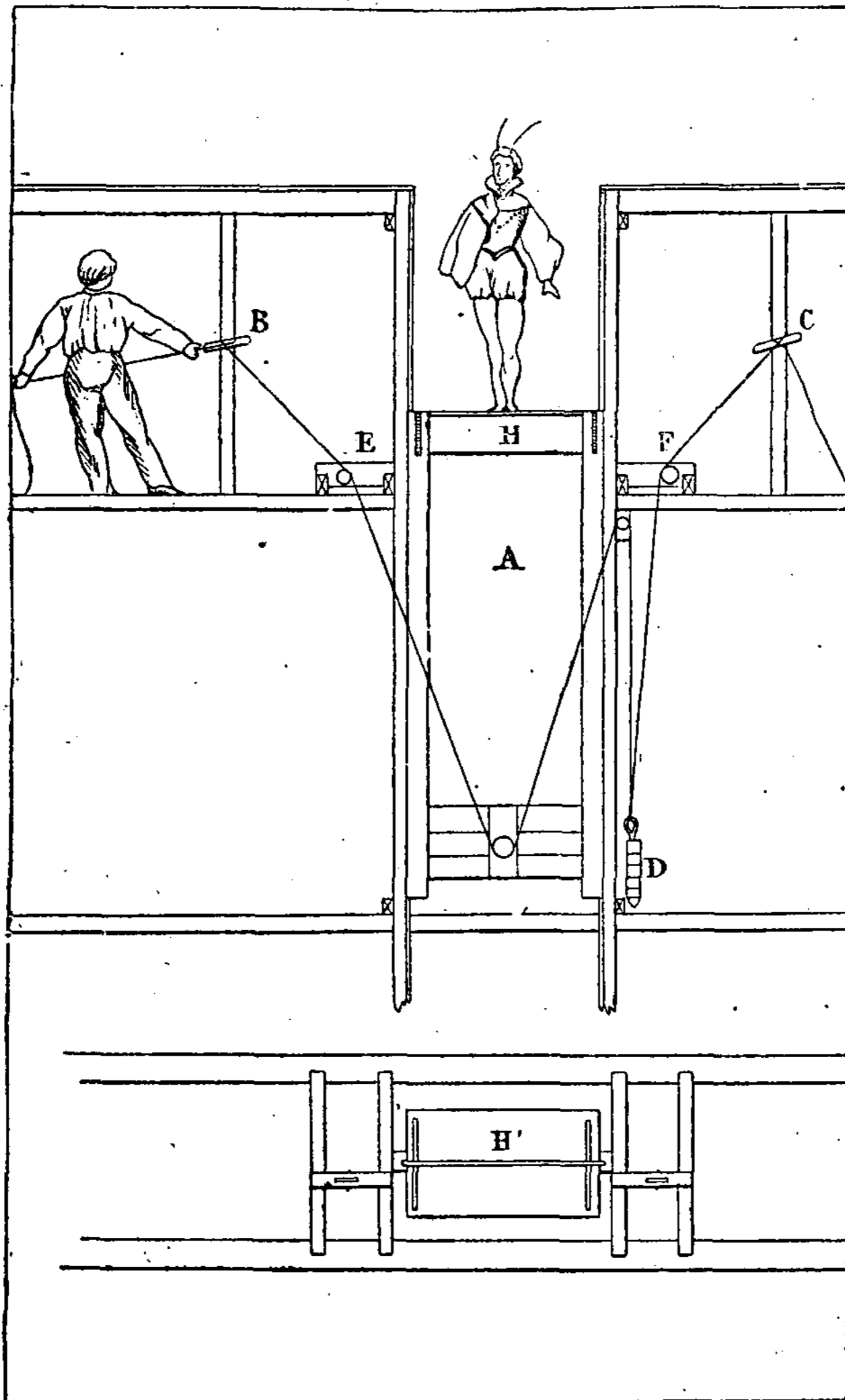
Fig. 9. — Équipe d'une trappe.
