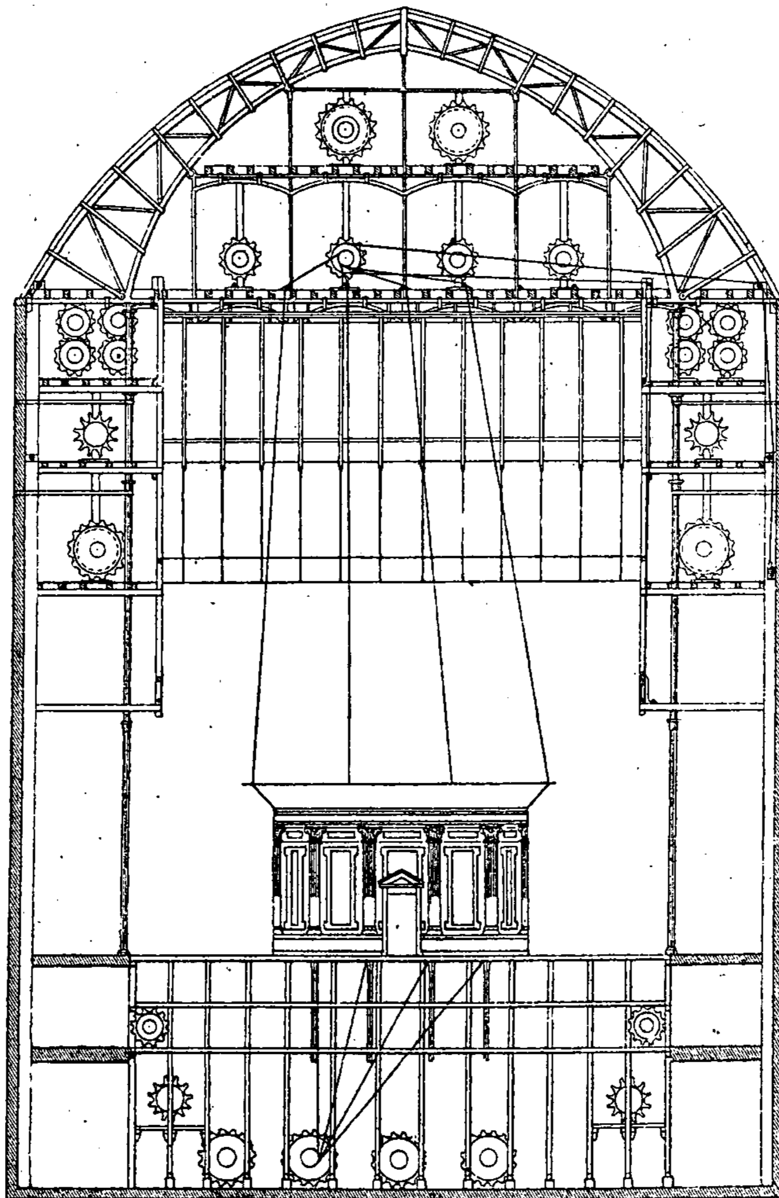
Fig. 60. — Coupe transversale. (Une ferme et un plafond équipés.)
