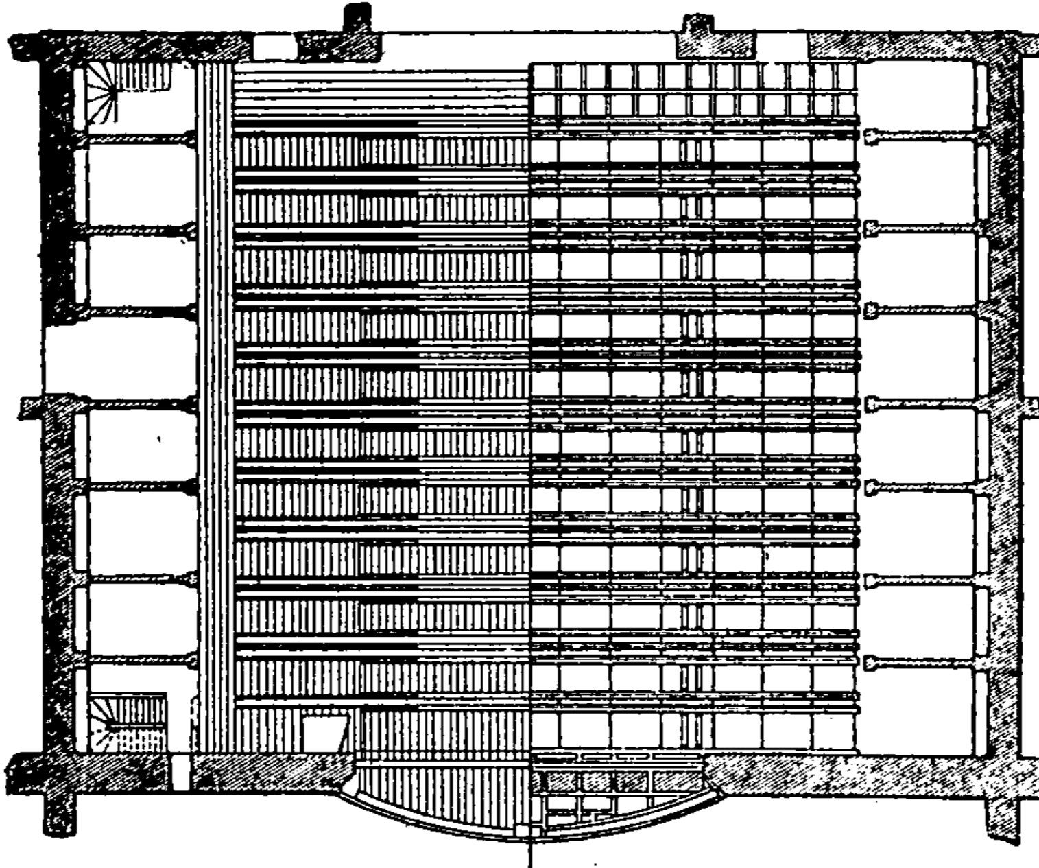
Fig. 5. — Plan d'un grand théâtre.
