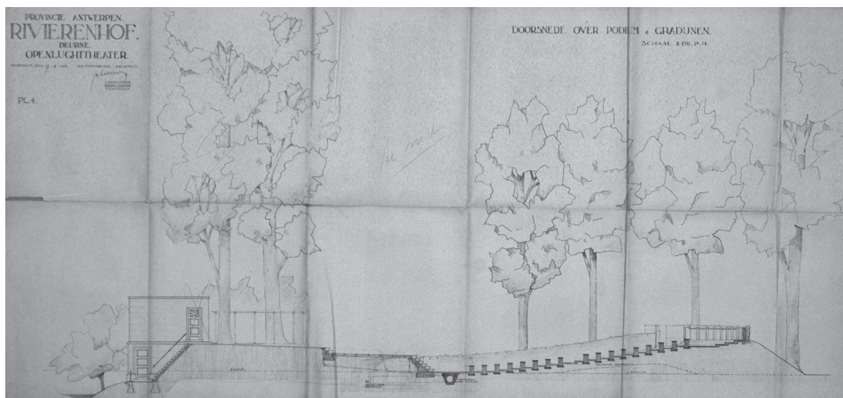
Afbeelding 3: Jozef Schellekens, Ontwerp voor het Openluchttheater Rivierenhof (voorlopig ontwerp; op dat ogenblik nog achter het kasteeltje gesitueerd) , 7 maart 1943. Bron: Provinciearchief Antwerpen.
